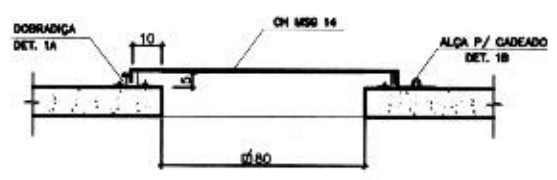
DETALHE 1 INSPEÇÃO
