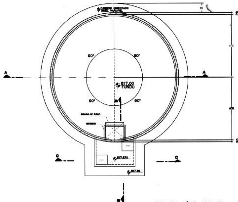
PLANTA NÍVEL 821.65 ESC.: 1:75
