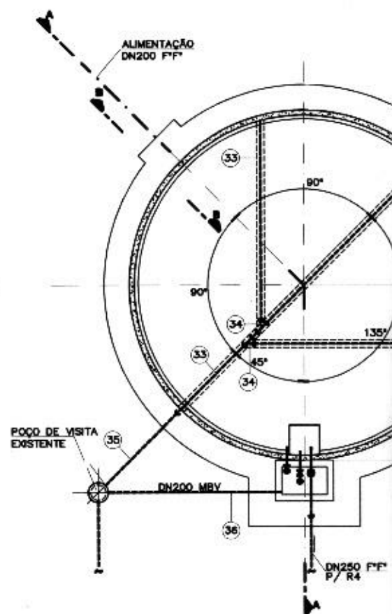
PLANTA NÍVEL 821.65 ESC.: 1:75
