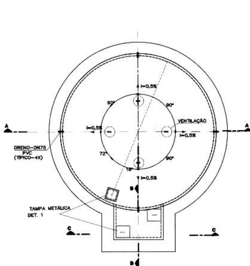
PLANTA COBERTURA ESC.: 1:75
